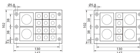
CES ET double row cable entry frame
