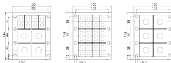
CES ET Triple row cable entry frame
