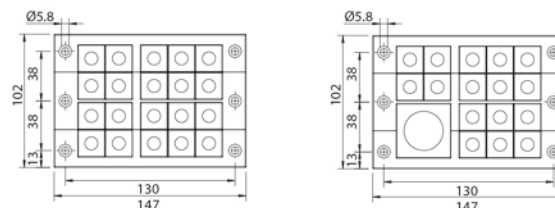
CES ET double row cable entry frame
