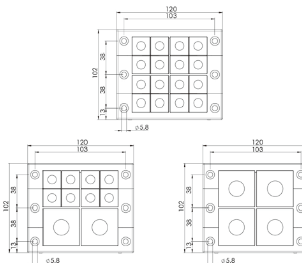
CES ET double row cable entry frame
