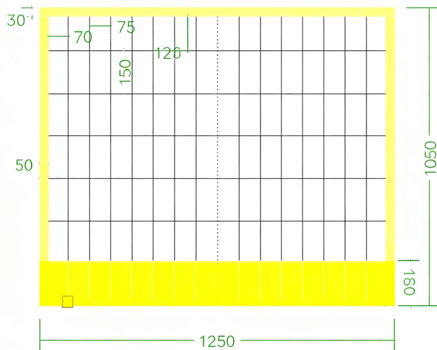
Edge guardrail drawing
