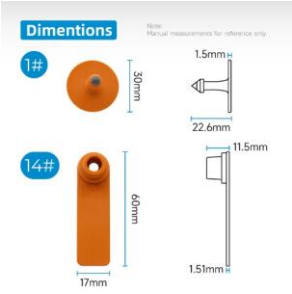
ITEM-11 Goat/Lamb Ear Tag: 1# + 14#
