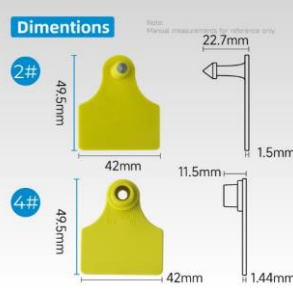
ITEM-8 Pig/Goat Ear Tag: 2#+4#
