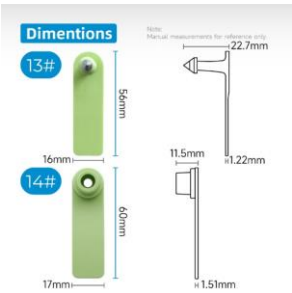
ITEM-13 Goat/Lamb Ear Tag: 13# + 14#
