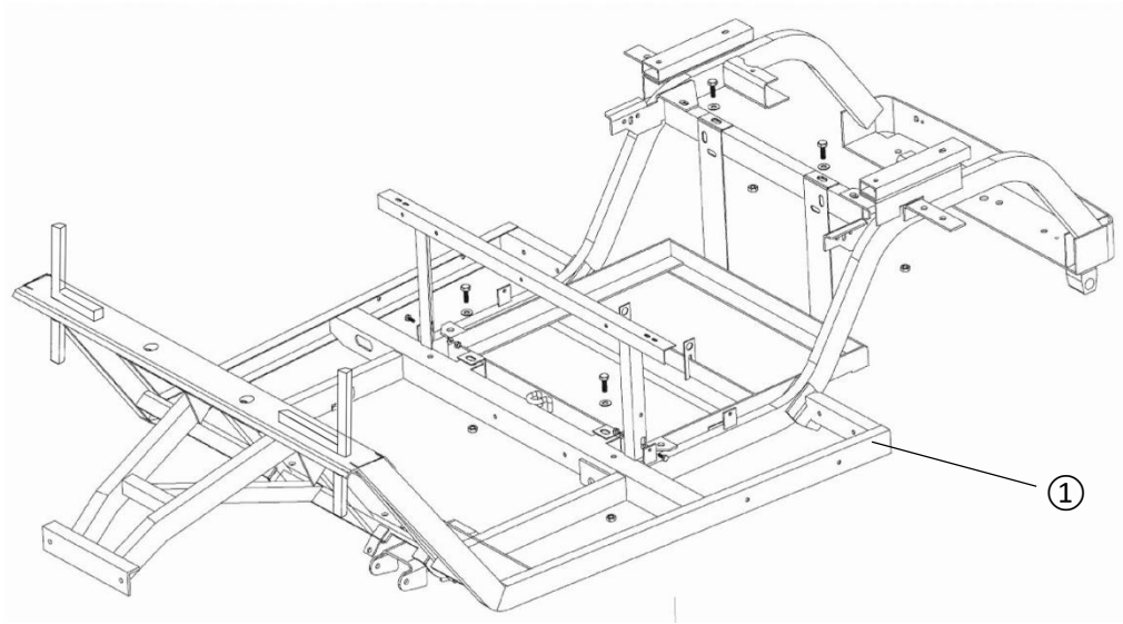
1.1 Frame (CA 底盘总成)
