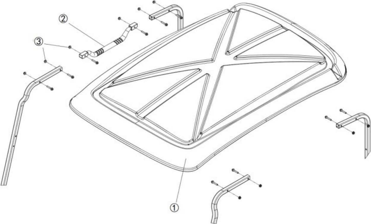
3.8.2 2P Roof (2 座顶棚总成)
