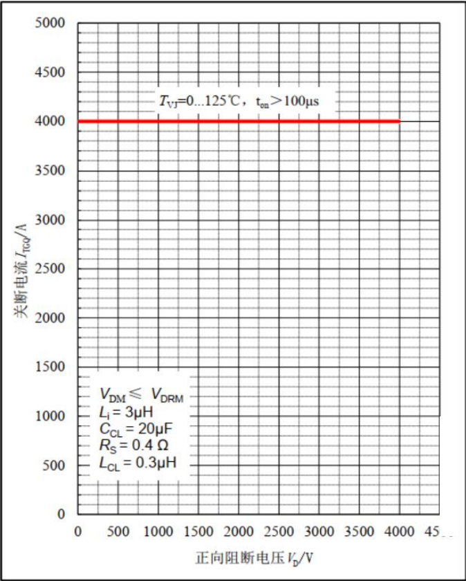
图3. 安全工作区
