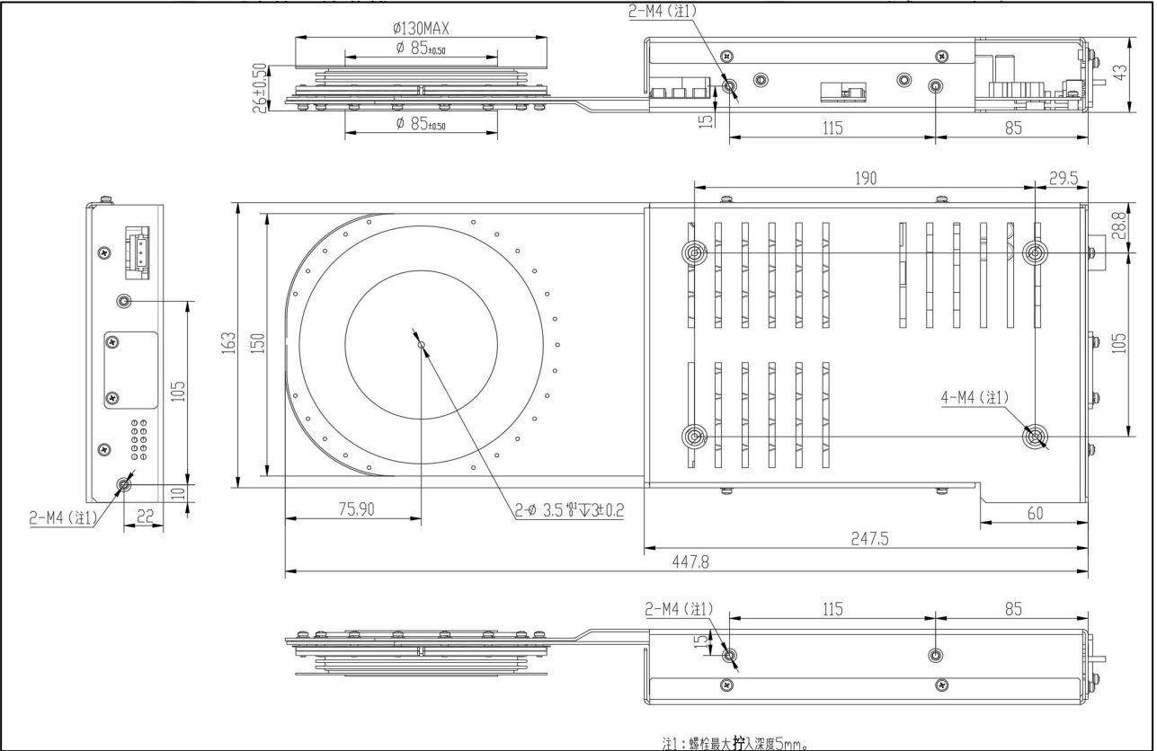
图7. IGCT器件外形图 (单位: mm)
