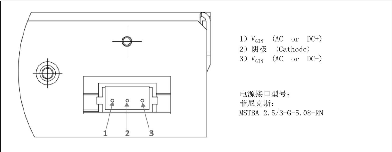
图8. 门极单元电源接口引脚图
