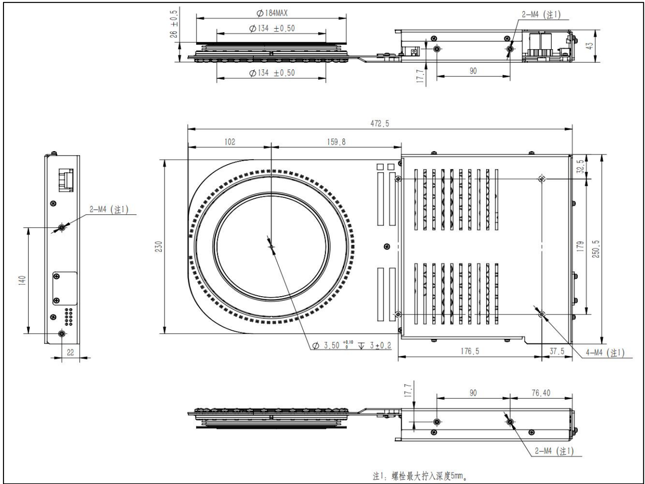
图6. IGCT器件外形图（单位：mm）
