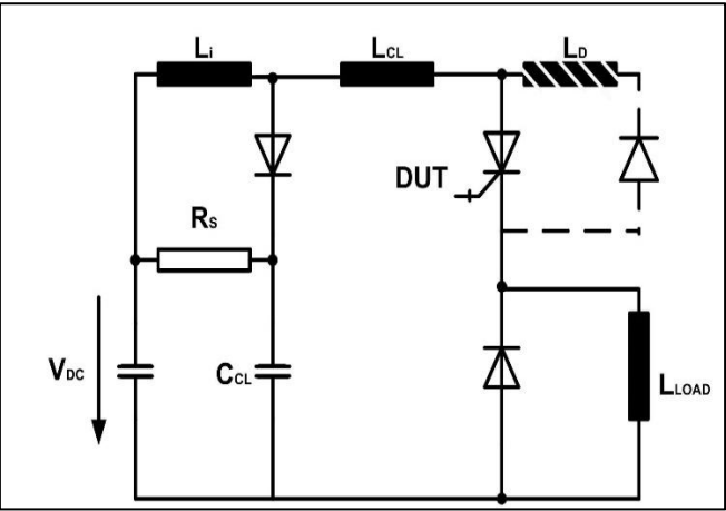
图5. IGCT测试原理电路
