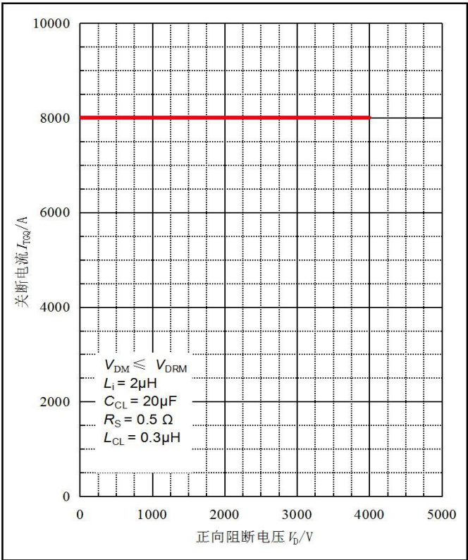
图3. 安全工作区
