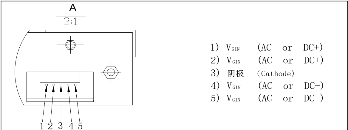
图7. 门极单元电源接口引脚图
