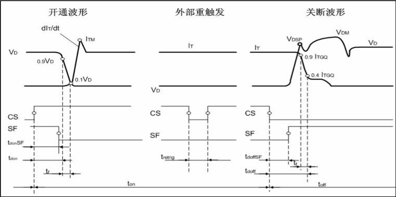
图8. IGCT器件电压电流波形
