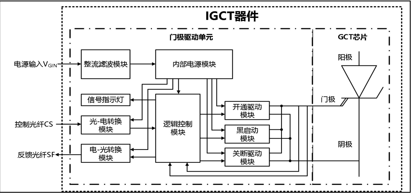
图9. IGCT器件门极电路框图
