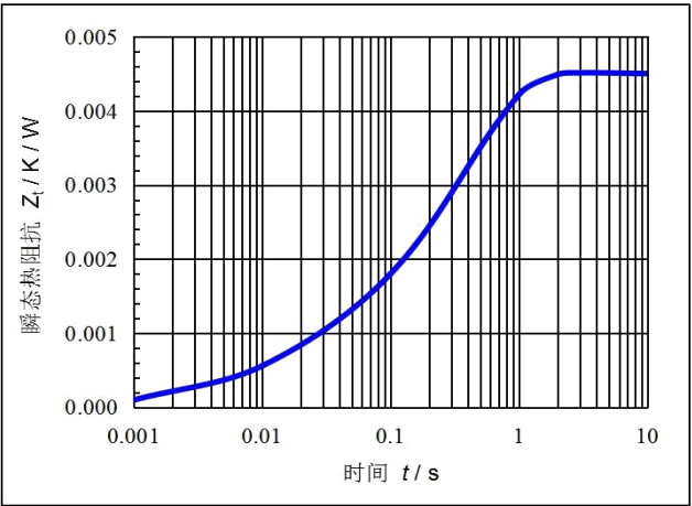
图4. 瞬态热阻抗曲线
