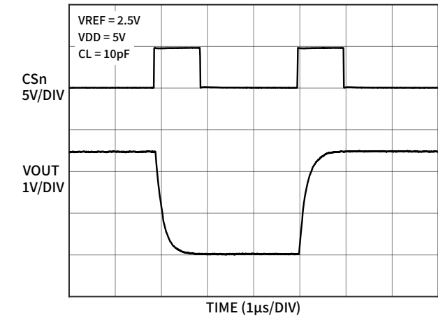
图 16 满量程高低电平转换
