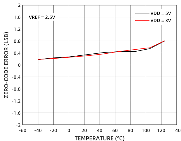
图 13 零码输入误差的温度特性
