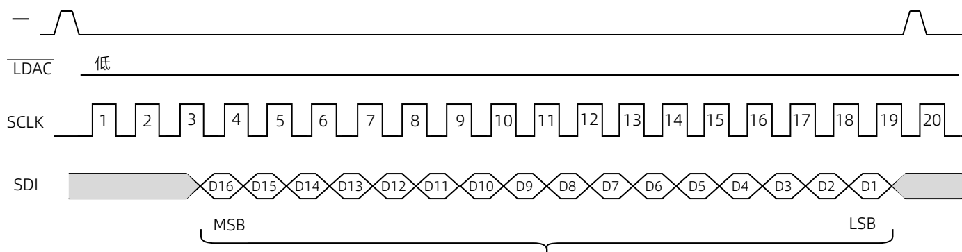
图 19 时序图
