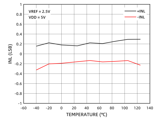
图 4 INL 的温度特性 (5V)
