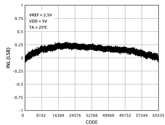
图 2 INL
