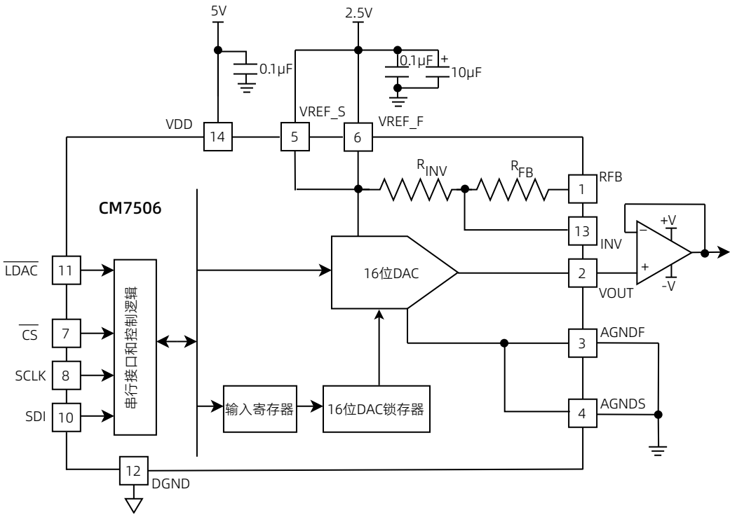
图 20 典型连接
