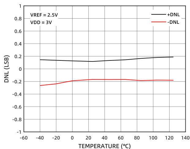
图 9 DNL 的温度特性 (3V)
