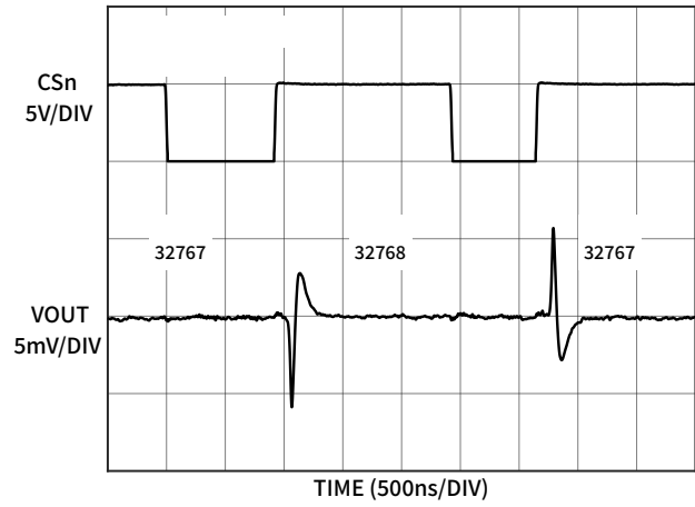
图 17 主进位翻转毛刺脉冲
