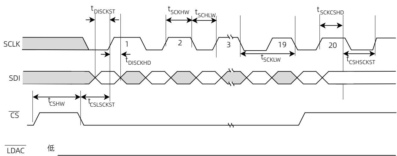
图 1 SPI 时序图
