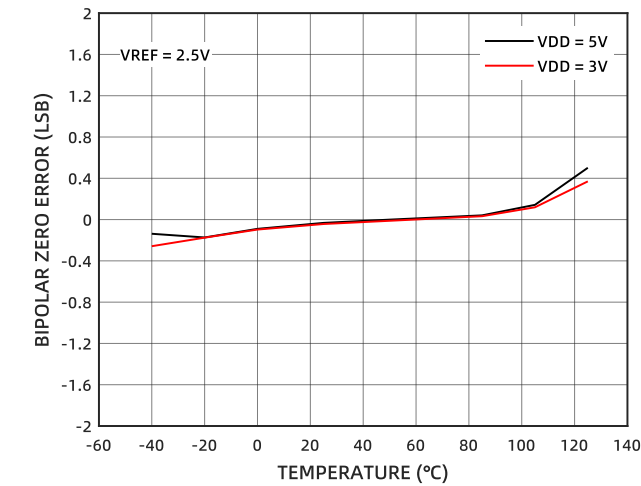
图 14 双极性零压失调误差的温度特性
