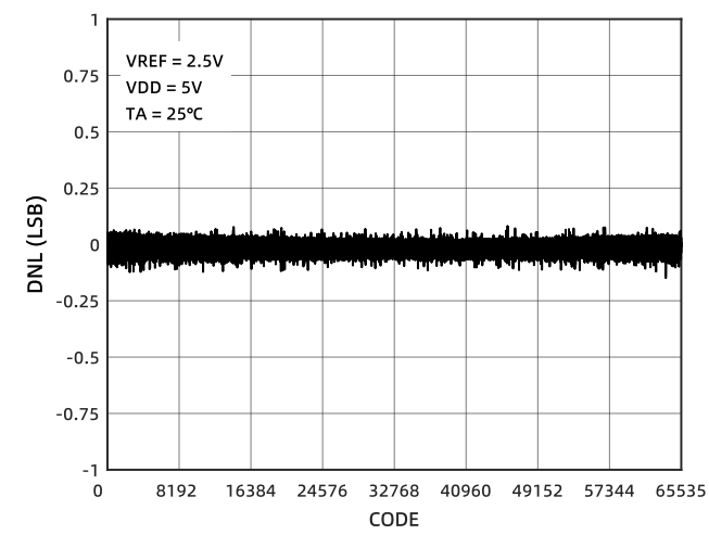
图 6 DNL
