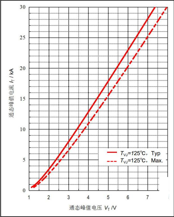
图2. 大电流下通态伏安特性
