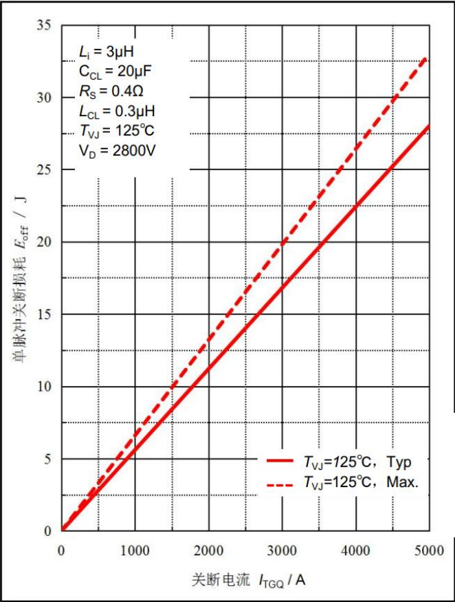
图3. 单脉冲关断能量与关断电流的关系曲线
