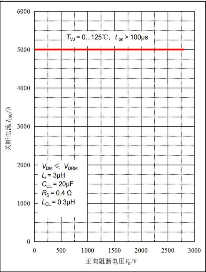
图4. 安全工作区
