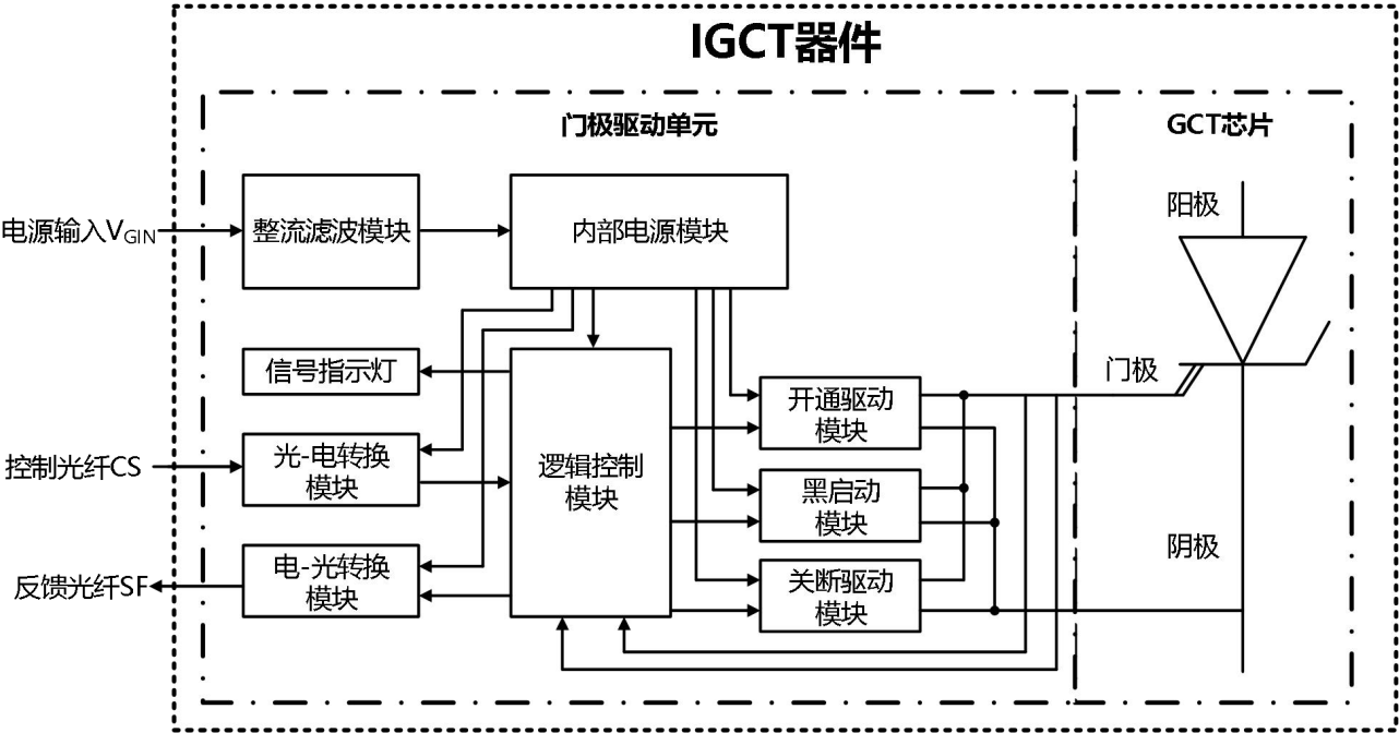
图12. IGCT器件门极电路框图
