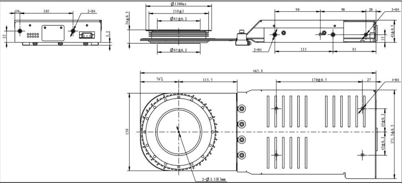
图10. IGCT器件外形图（单位：mm）
