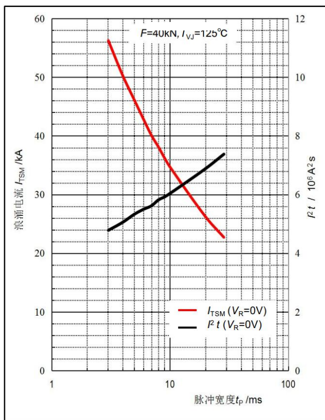
图5. 浪涌电流与正弦半波脉冲宽度关系
