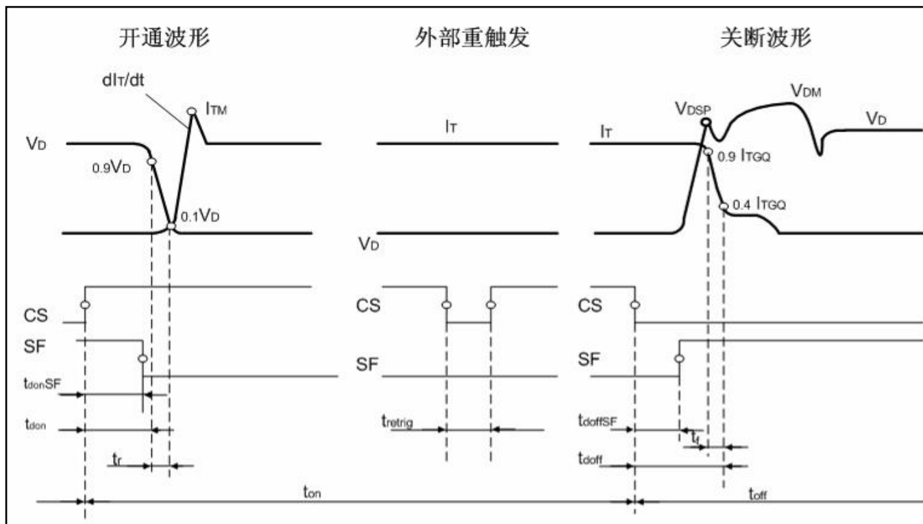
图7. IGCT器件电压电流波形
